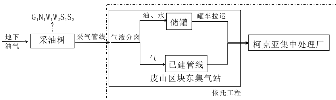
图 3.3-4 井场油气开采及集输工艺流程图
